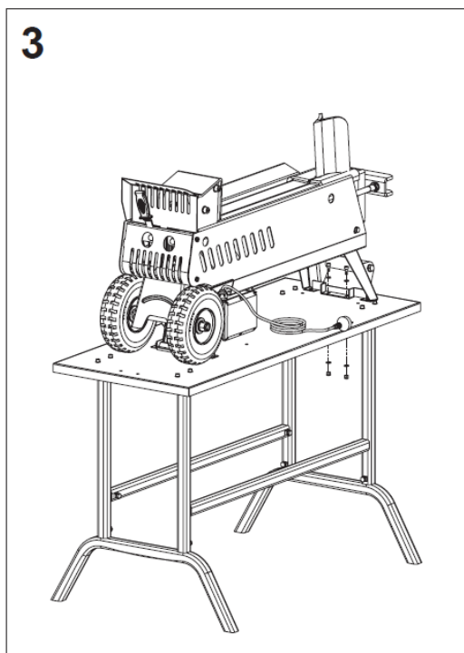
Рисунок 1. Загальний вигляд виробів та схема складання..
