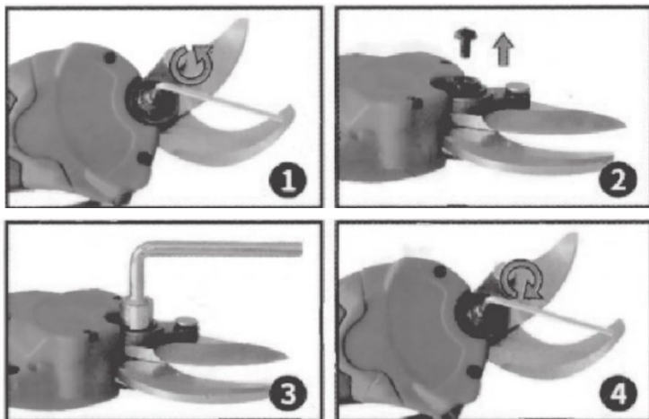
Рисунок. 7. Усунення зазору між лезами ножів.
