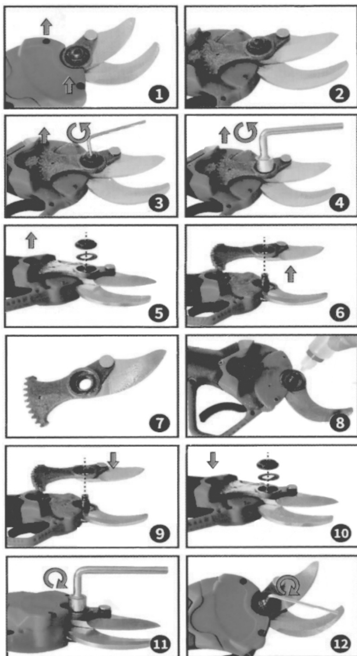
Рисунок. 8. Заміна та змащування ножів.
