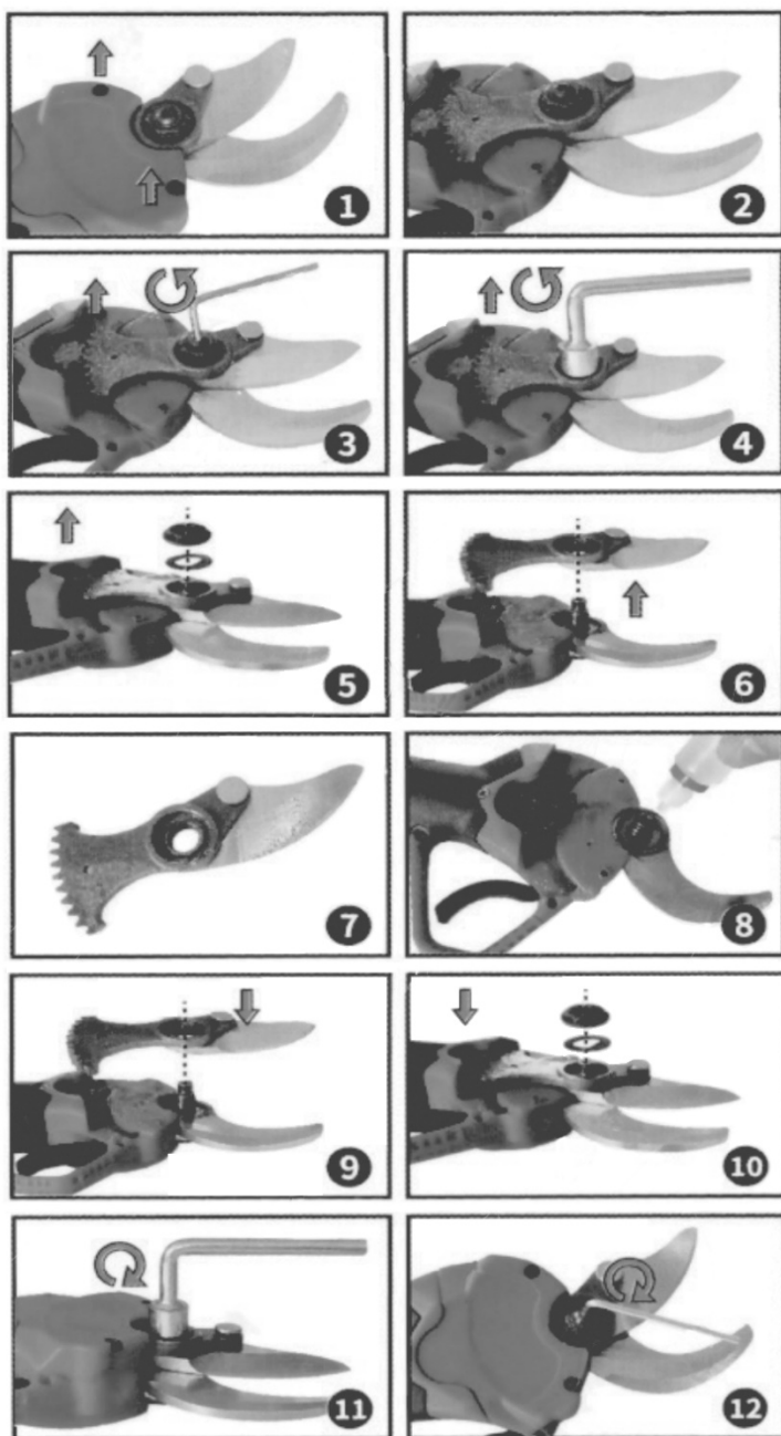
Рисунок. 7. Заміна та змащування ножів.
