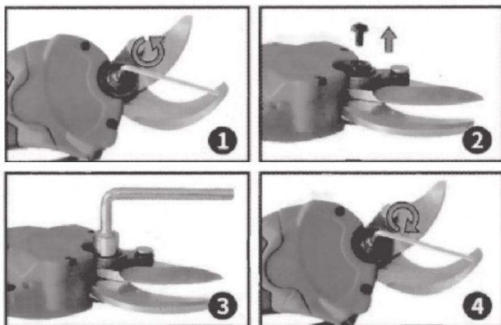
Рисунок. 6. Усунення зазору між лезами ножів.
