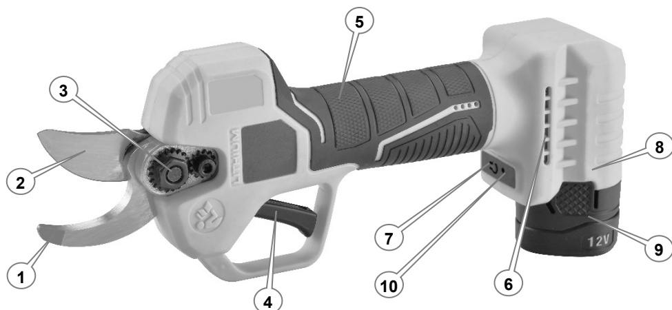
Рисунок 1. Загальний вигляд виробу.
