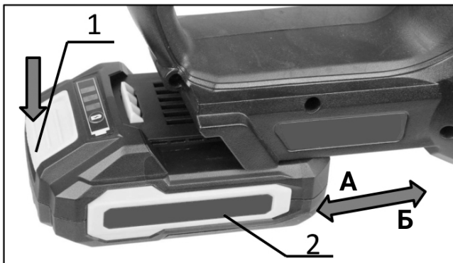
Рисунок 3. Схема встановлення (зняття) акумуляторної батареї.
