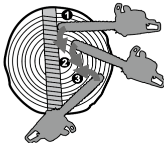
Рисунок 14. Схема розпилювання колоди з використанням зубчастого упору електричної пили.
