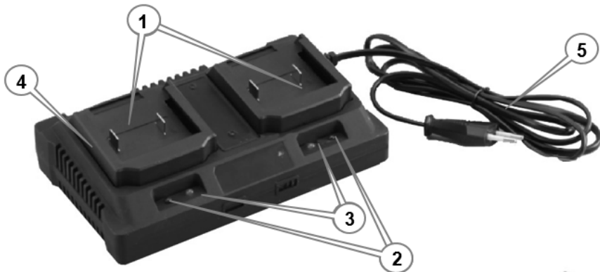
Рисунок 3. Загальний вигляд зарядного пристрою (модель «1820c double», ТМ «Vitals»).
