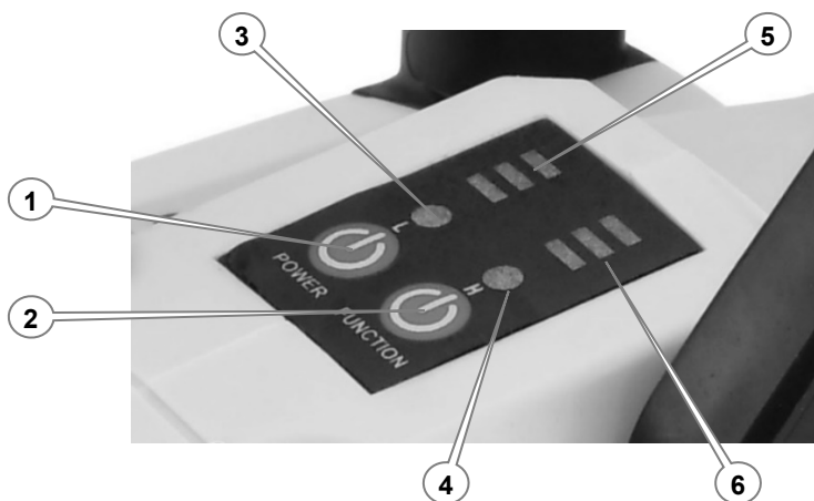
Рисунок 2. Загальний вигляд контрольної панелі.
