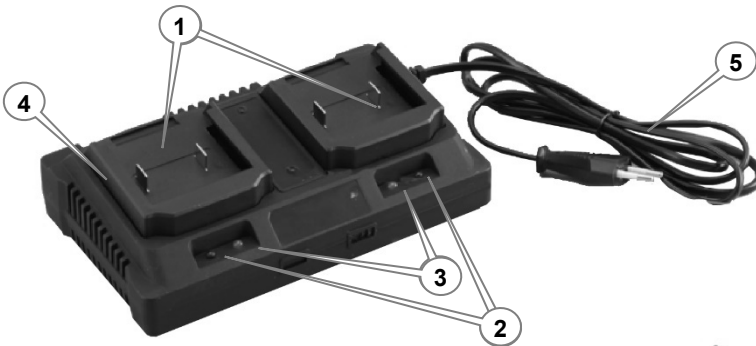
Рисунок 4. Загальний вигляд зарядного пристрою (модель «1820c double», ТМ «Vitals»).
