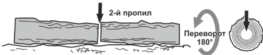
Рисунок 14. Схема остаточного розпилу колоди з протилежного боку.
