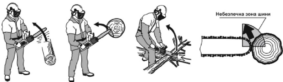
Рисунок 5. Приклади виникнення небезпечної віддачі виробу.
