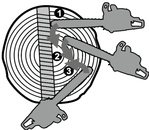
Рисунок 17. Схема розпилювання колоди з використанням зубчастого упору електропили.
