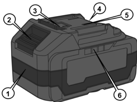
Рисунок 2. Загальний вигляд акумуляторної батареї (модель «ASL 1840ns-10C Type-c», ТМ «Vitals»).
