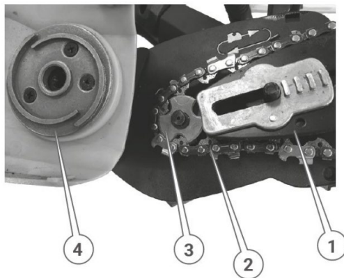
Рисунок 5. Схема встановлення різального блока: направної шини та ланцюга.
