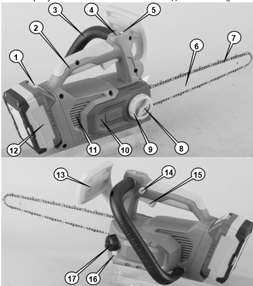
Рисунок 1. Загальний вигляд виробу.
