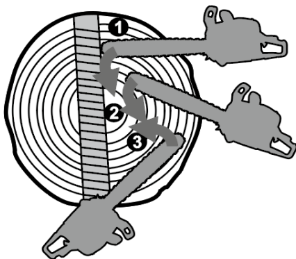
Рисунок 14. Схема розпилювання колоди з використанням зубчастого упору електропили.
