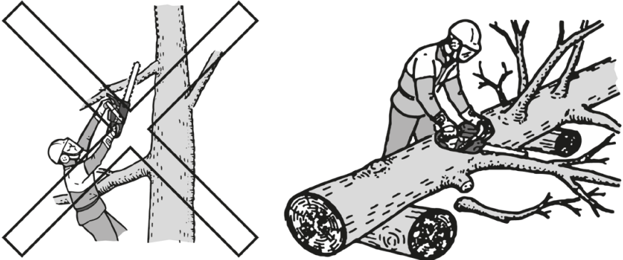
Рисунок 13. Схема обрізання малих гілок.
