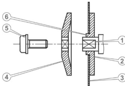
Рисунок 2. Встановлення циркулярного диска.
