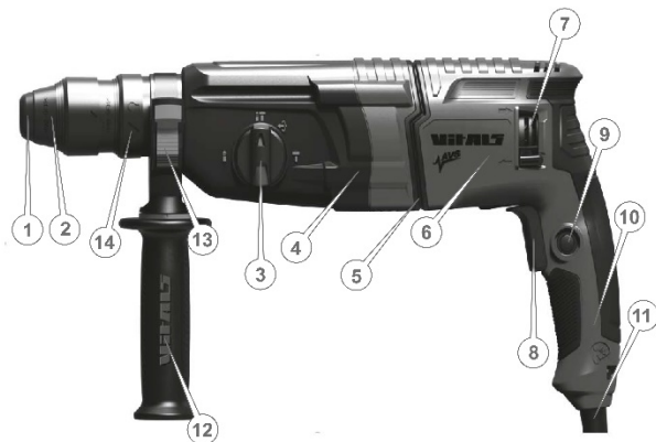
Рисунок 1. Загальний вигляд конструкції.
