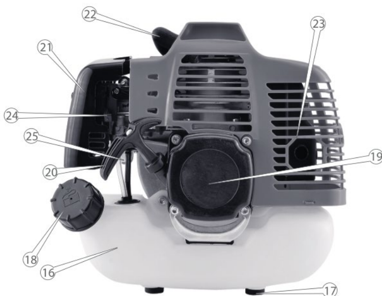
Рисунок 1. Загальний вигляд мотокози ТМ «Vitals», моделі «ВК 521п».
