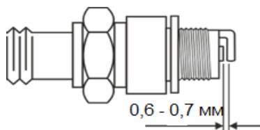
Рисунок 17. Свічка запалювання. Рекомендований зазор між електродами.
