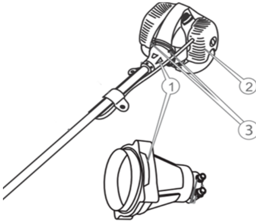
Рисунок 2. Схема приєднання «штанги» до двигуна виробу.
