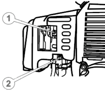
Рисунок 18. Схема розташування гвинтів регулювання карбюратора.
