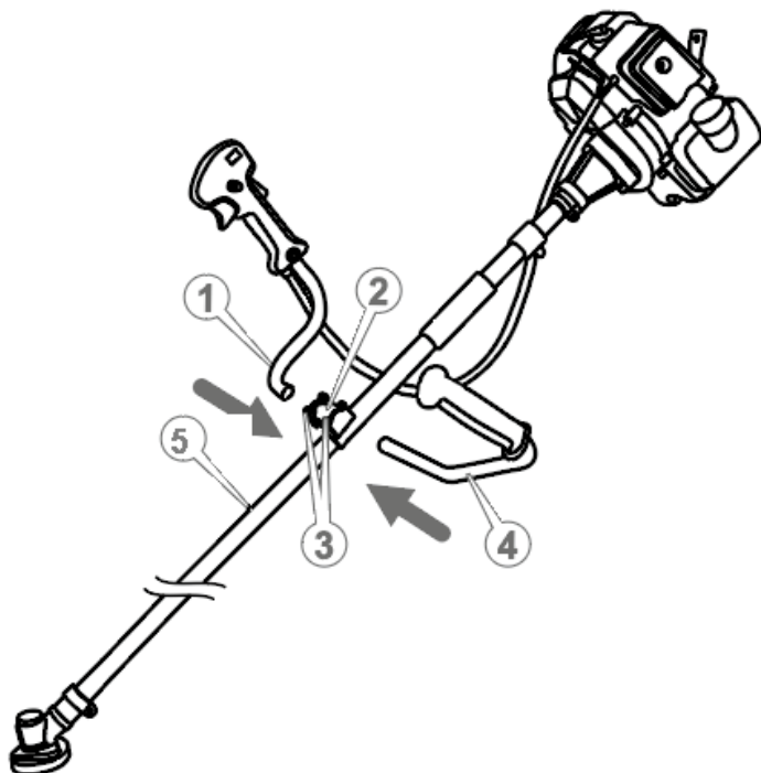
Рисунок 2. Схема встановлення руків'їв виробу.
