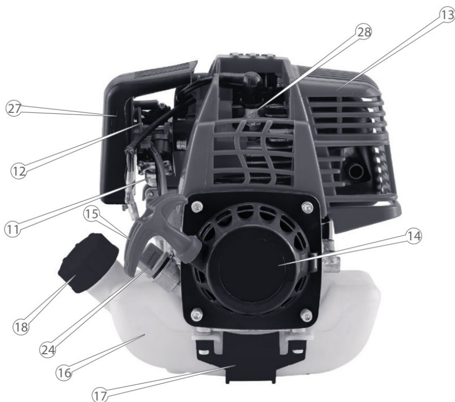
Рисунок 1. Загальний вигляд мотокози ТМ «Vitals», моделі «BK 3110-4n».
