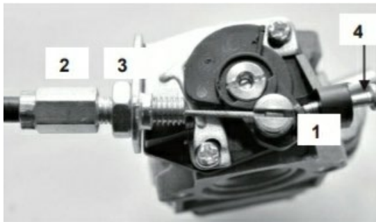
Рисунок 8. Схема під'єднання тросика дроселя.
