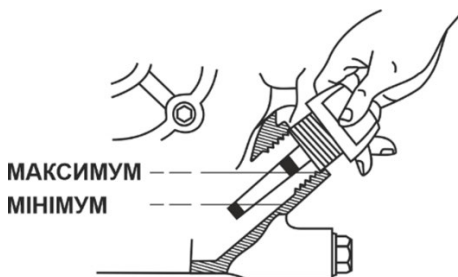
Рисунок 10. Перевірка рівня мастила в картері двигуна.
