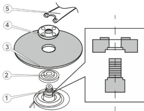
Рисунок 2. Схема встановлення та зняття абразивного диска.
