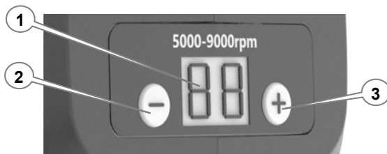
Рисунок 2. Загальний вигляд панелі керування режимом швидкості.
