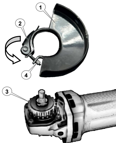
Рисунок 5. Встановлення захисного кожуха.
