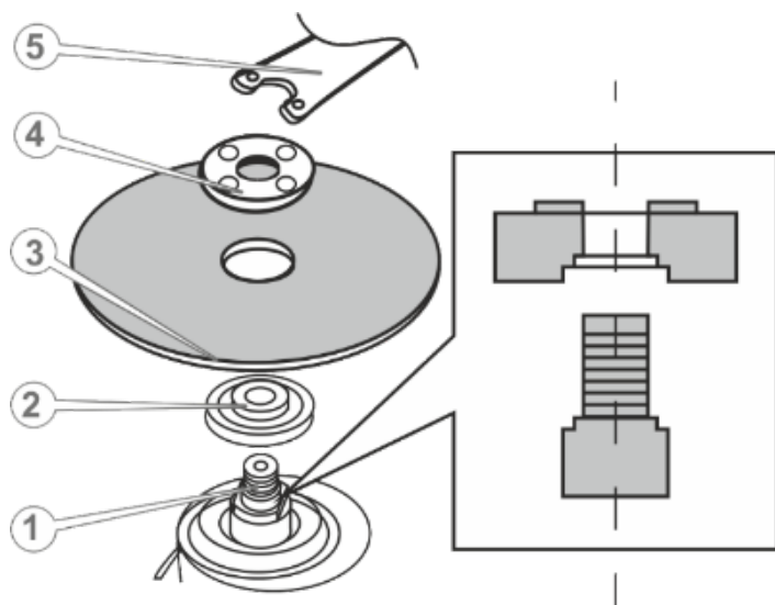
Рисунок 7. Схема встановлення та зняття абразивного диска.
