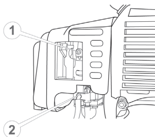
Рисунок 17. Схема розташування гвинтів регулювання карбюратора.
