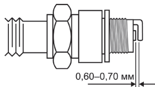
Рисунок 16. Свічка запалювання. Рекомендований зазор між електродами.
