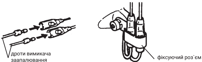
Рисунок 9. Схема під'єднання дротів вимикача запалювання.
