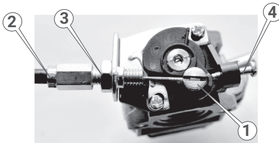
Рисунок 8. Схема під'єднання тросика дроселя.
