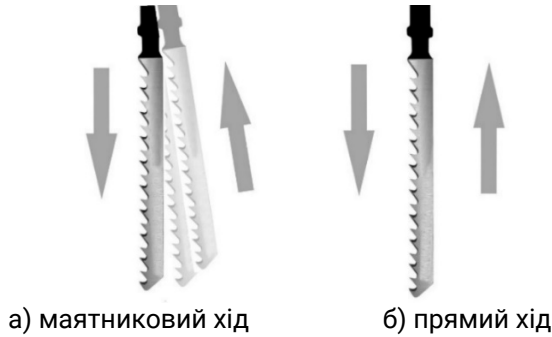
Рисунок 4. Види руху пилки.
