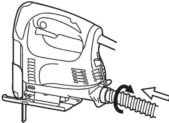
Рисунок 5. Схема під'єднання системи пиловідведення або пилосямока до виробу.
