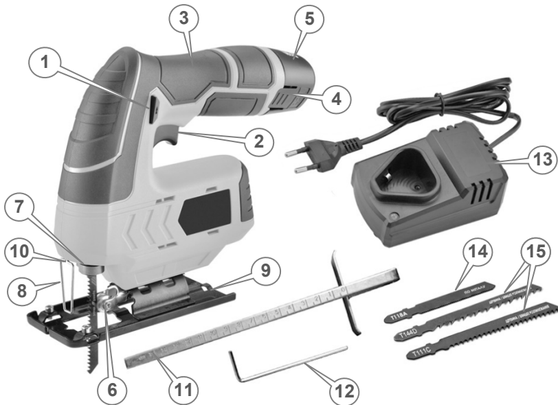
Рисунок 1. Загальний вигляд моделі Ef 1265c Kit.
