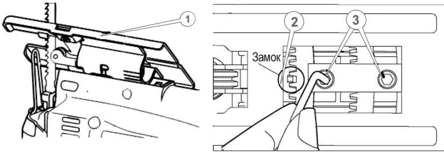
Рисунок 4. Схема налаштування кута різання до вертикалі.
