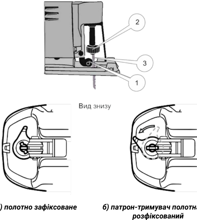
Рисунок 2. Схема встановлення різального полотна.
