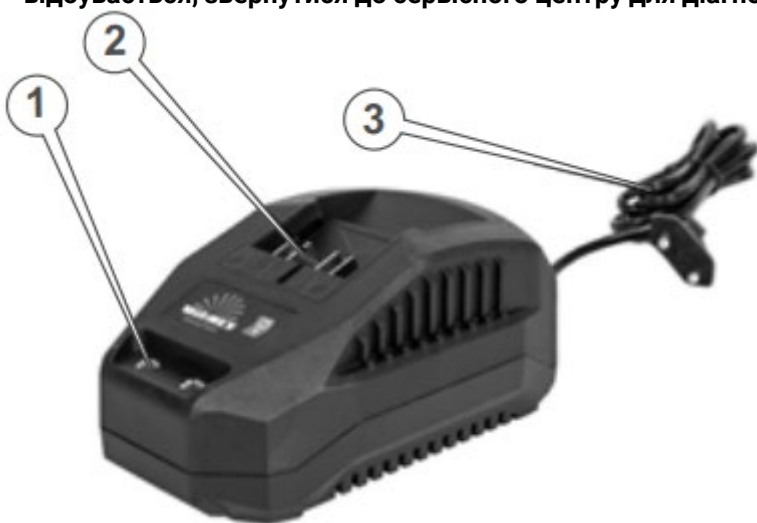
Рисунок 3. Загальний вигляд зарядного пристрою.
