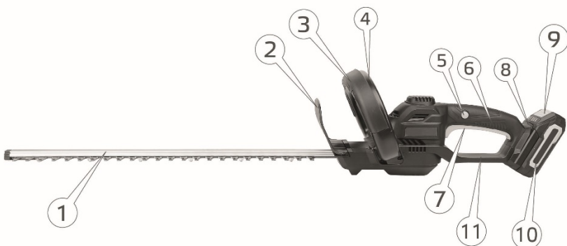
Рисунок 1. Загальний вигляд виробу.
