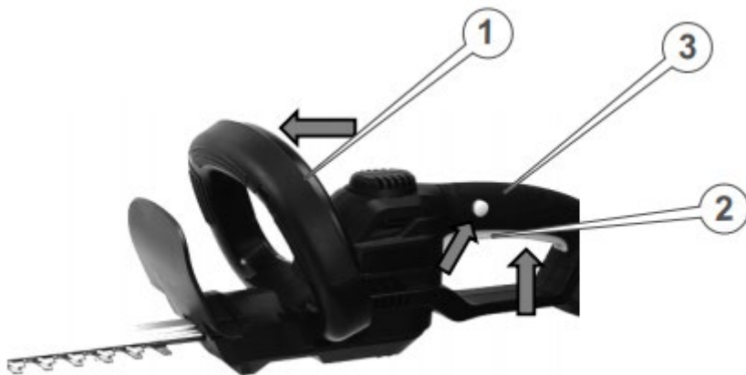
Рисунок 5. Схема запуску кущоріза.
