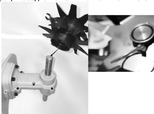
Рисунок 7. Схема встановлення та фіксації робочої насадки.
