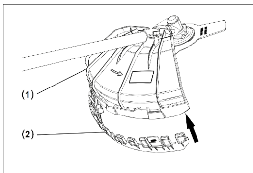
Рисунок 6. Схема встановлення захисного кожуха на «штангу».
