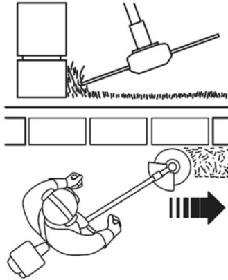
Рисунок 14. Схема скошування трави вздовж перешкод.
