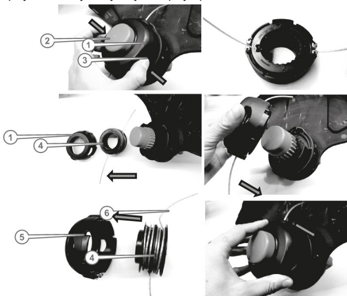
Рисунок 17. Схема заміни жилки різальної головки.
