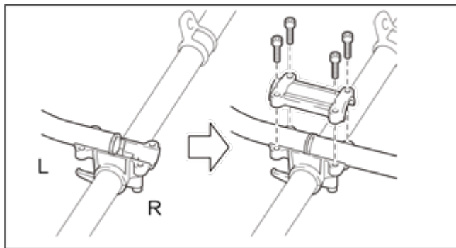
Рисунок 3. Схема встановлення частин руків'я на «штангу» коси.
