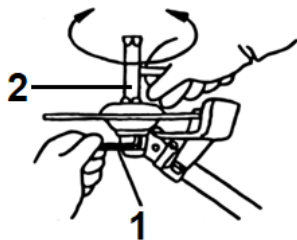
Рисунок 7. Схема встановлення дискового різального ножа.
