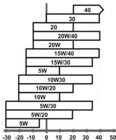
Рисунок 3. Залежність в'язкості мастила від температури сезону.
