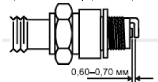
Рисунок 2. Свічка запалювання. Рекомендований зазор між електродами.
