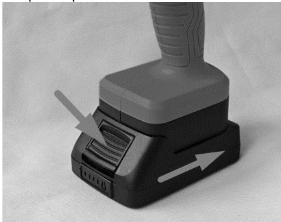
Рисунок 4. Схема встановлення/зняття АКБ.
