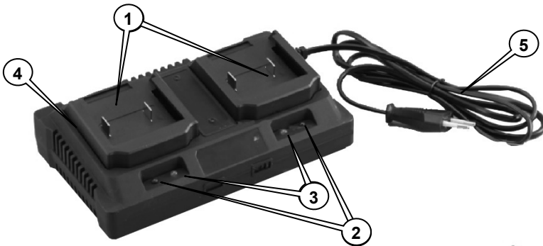
Рисунок 3. Загальний вигляд зарядного пристрою (модель «1820n double», ТМ «Vitals»).
