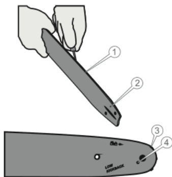
Рисунок 17. Обслуговування «шини»
