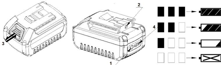
Рисунок 7. Акумуляторна батарея.
