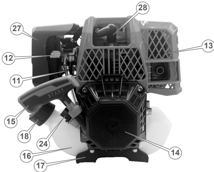
Рисунок 1. Загальний вигляд виробу.
