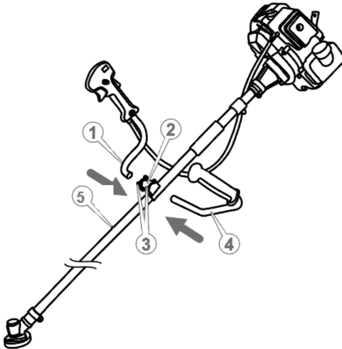
Рисунок 3. Схема встановлення руків'їв виробу.
