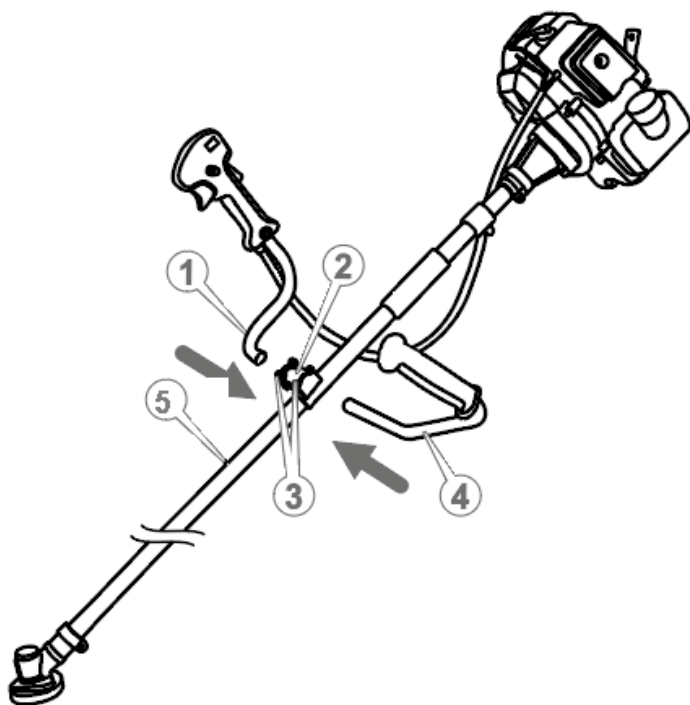
Рисунок 2. Схема встановлення руків'їв в роботу.
