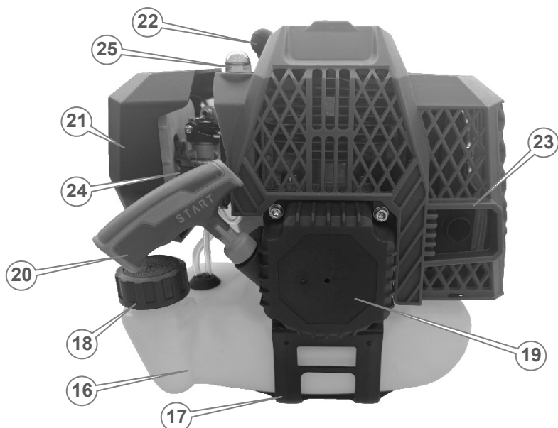
Рисунок 1. Загальний вигляд мотокоши моделі «BK 523n».
