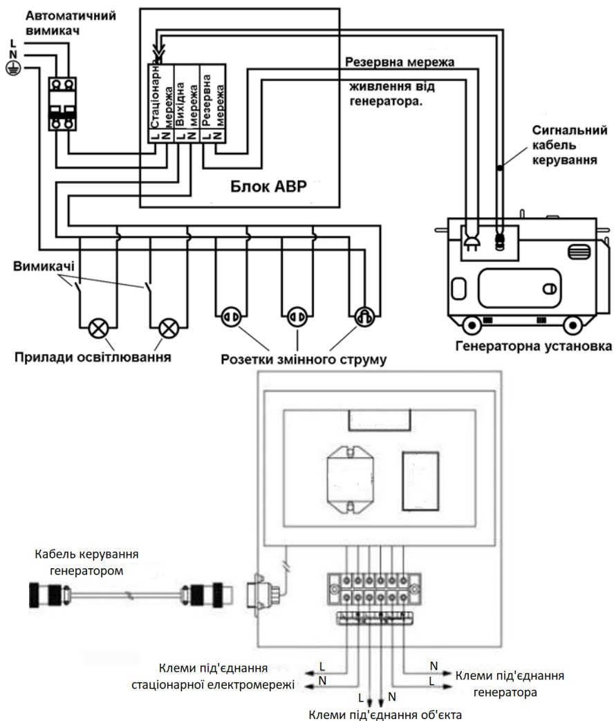
а) електрична схема під'єднання блока АВР (ATS) до 1-фазної електромережі.
