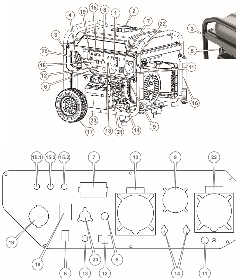
Рисунок 1. Загальний вигляд виробу та панелі керування.
