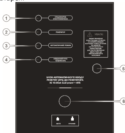
Рисунок 2. Загальний вигляд передньої панелі блоку аварійного вводу резерву (ATS).
