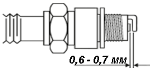
Рисунок 7. Величина зазору між електродами свічки запалювання.
