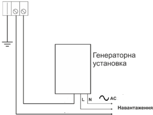
Рисунок 5. Схема заземлення виробу.
