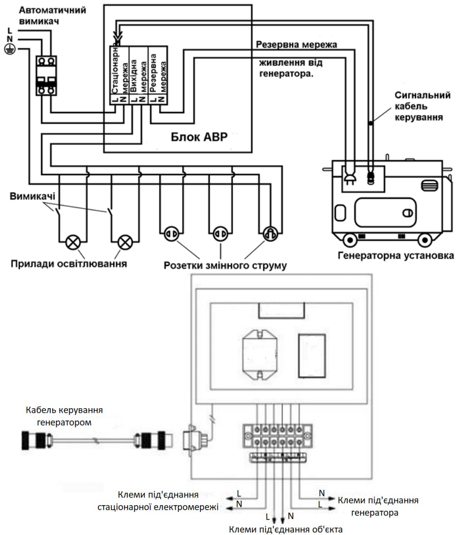
а) електрична схема під'єднання блока АВР (АТЗ) до 1-фазної електромережі.
