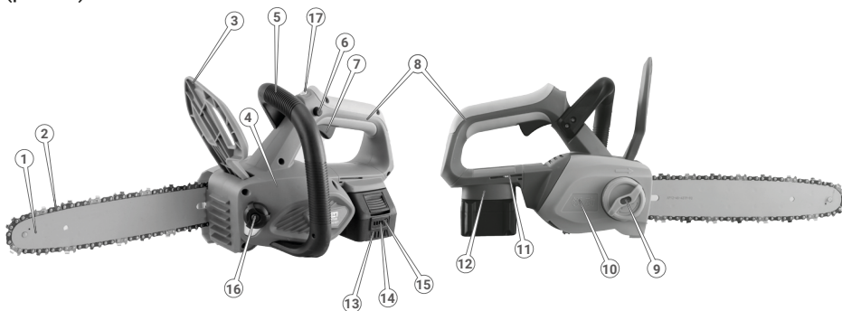
Рисунок 1. Загальний вигляд основних компонентів виробу.
