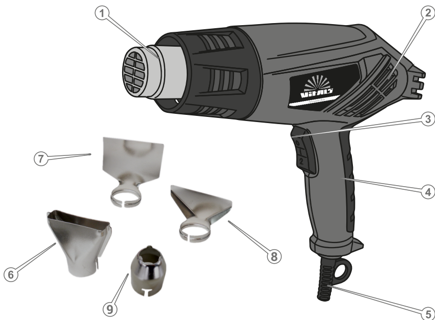
Рисунок 1. Загальний вид виробу та насадок.
